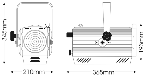
Cetra f100 LED RGBW
